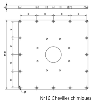
CONTREPLAQUE Z2
